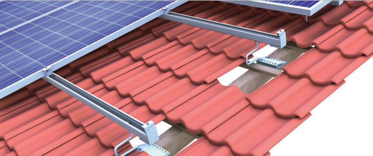
novotegra top-fix – etlags-klemmesystem med moduler monteret på højkant
